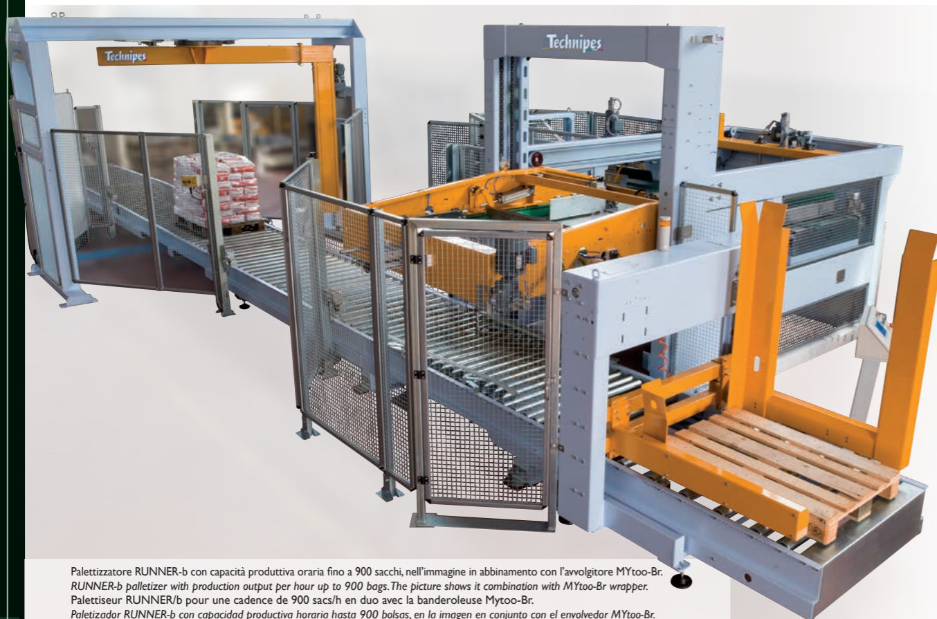
Rulliera di scarico del bancale finito Unloading roller conveyor of filled pallet. Convoyeur d'évacuation de la palette pleine Mesa de rodillos de descarga del palet terminado
